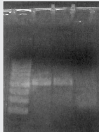
Abb. 15: Das Gelbild zeigt links den Marker. Die dickere Bande ist die 500-Basenpaarbande. Die Spur rechts neben dem Marker trägt eine Positivkontrolle. Es handelt sich hier um das PCR-Produkt des Fadenwurms Caenorhabditis elegans bei 532 Basenpaaren, für den die Primer konstruiert sind. Die Spur rechts daneben zeigt das PCR-Produkt eines Moosnematoden auf derselben Höhe. Die Spur daneben zeigt die Negativkontrolle, die auch negativ ausfällt.
