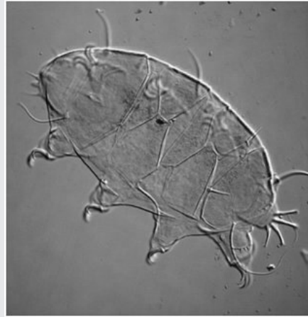
Abb. 16: Bärtierchen mit Platten ( Echiniscus testudo )
