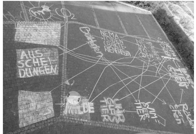
Abb. 8: Nahrungsnetz Moos auf dem Lehrerparkplatz des Marien-Gymnasiums in Werl
