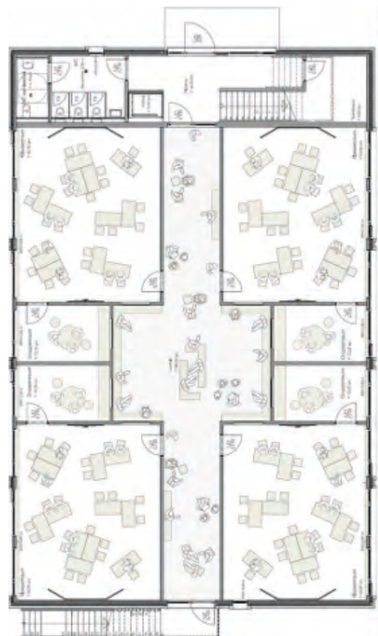
Abb.: Beispielhafte Innenraumaufteilung Hamburger Klassenhaus. Foto: SBH | Schulbau Hamburg
