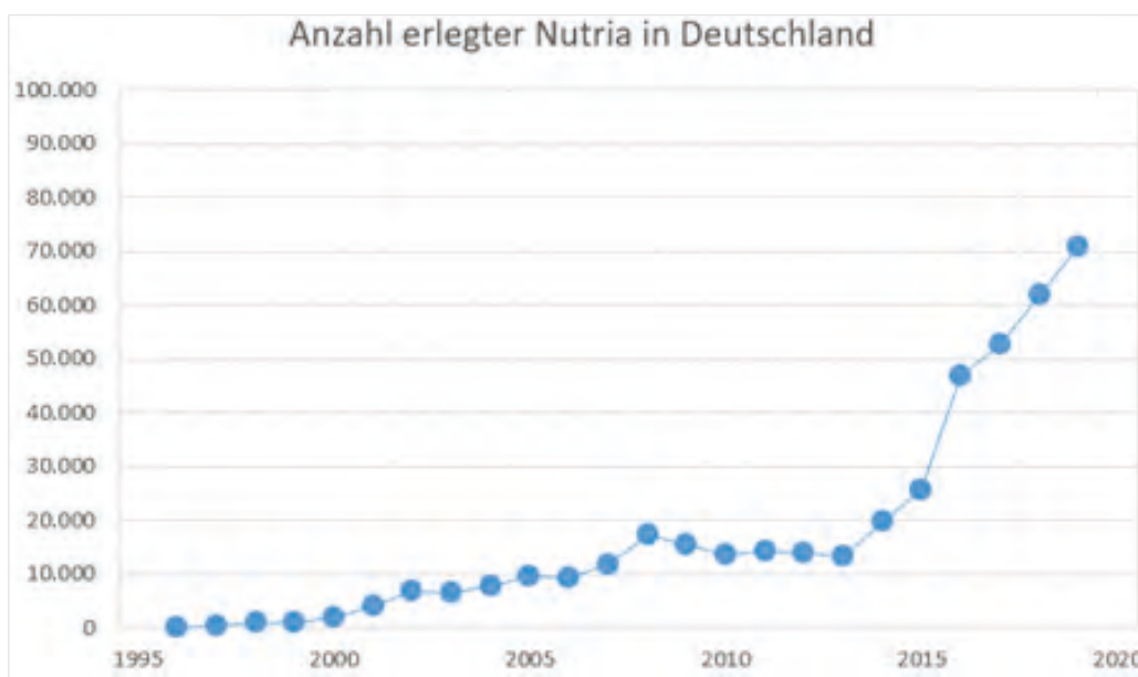
Abb. Grafik1: Anzahl erlegter Nutria in Deutschland. Aus: https://www.umweltanalysen.com/nutria/jagdstrecke/
